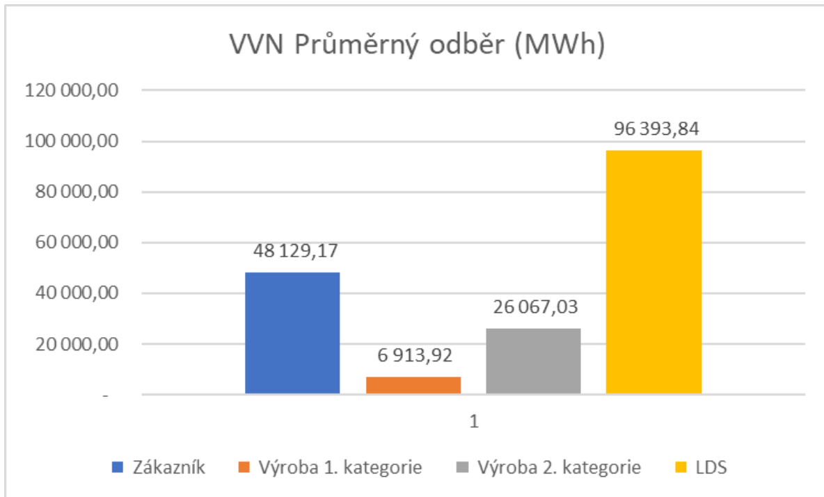
Obrázek 5 - Průměrný odběr jednotlivých kategorií VVN v roce 2020
