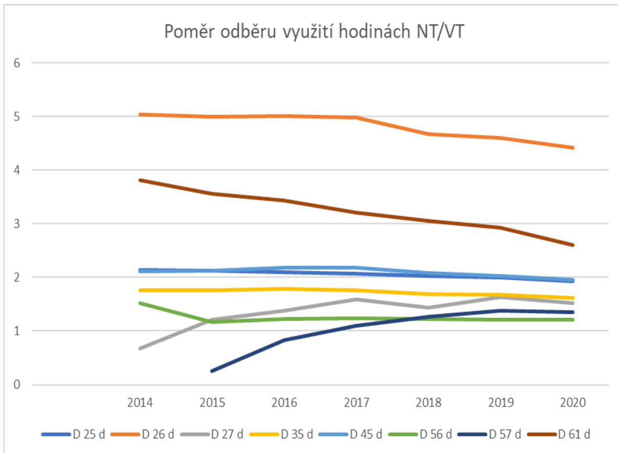
Obrázek 36 - Hodinové využití NT tarifu v porovnání s VT tarifem M00.
