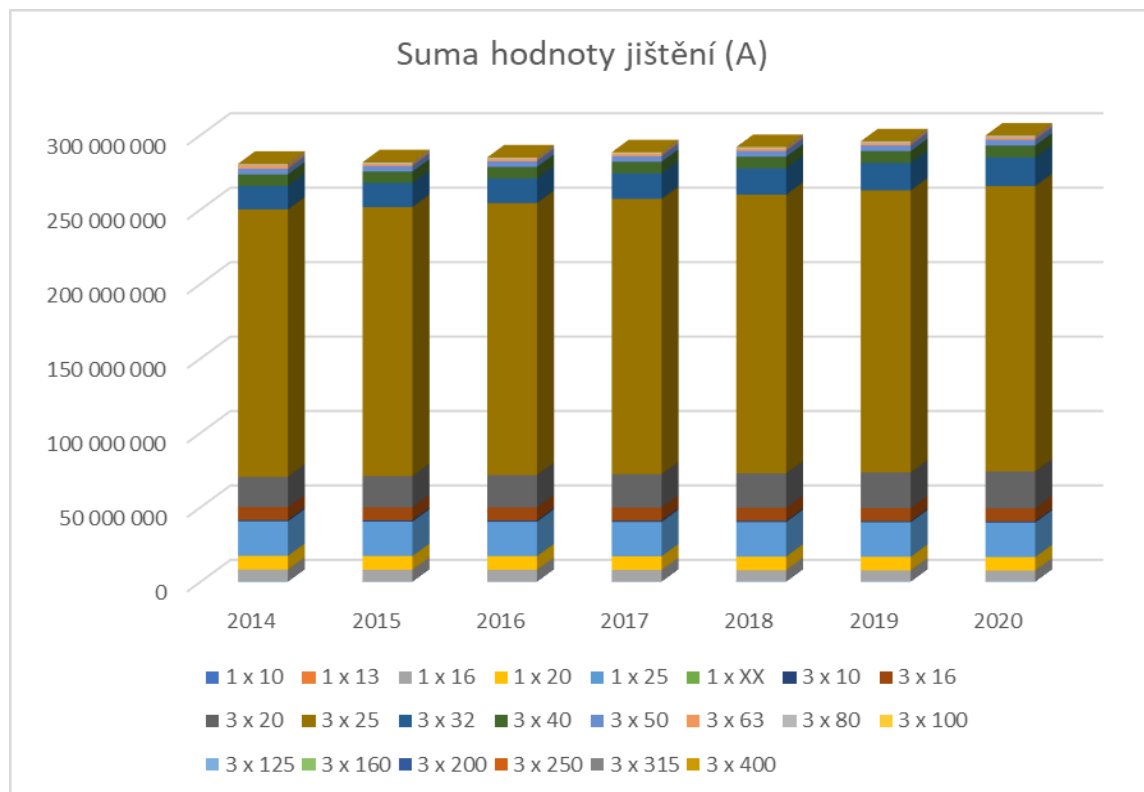
Obrázek 30 - Vývoj sumární hodnoty jistění MOO dle velikosti hlavního jističe
