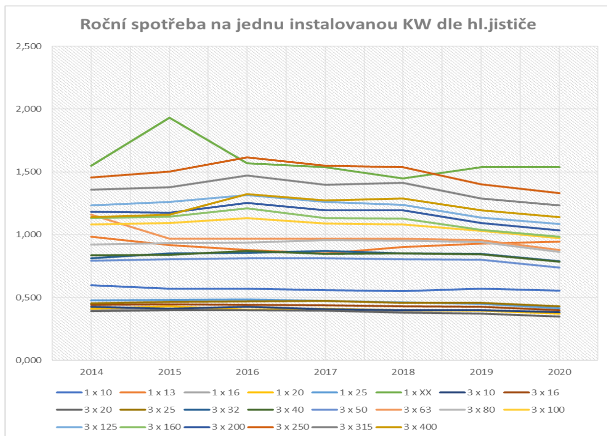
Obrázek 45 - Přehled využití kapacity hlavního jističe MOP přepočteného na jednu KW rezervovaného příkonu.
